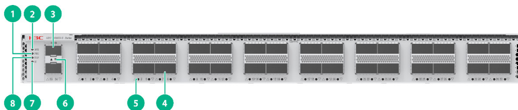
图2-6 S9600XP-32DH-G 前面板示意图
