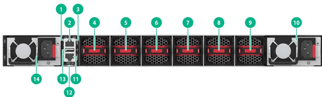
图2-7 S9600XP-32DH-G 后面板示意图
