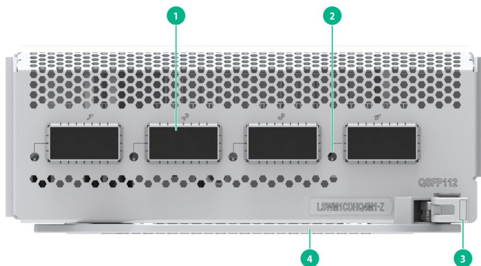
图4-3 LSWM1CDHQ4M1-Z 前面板示意图
