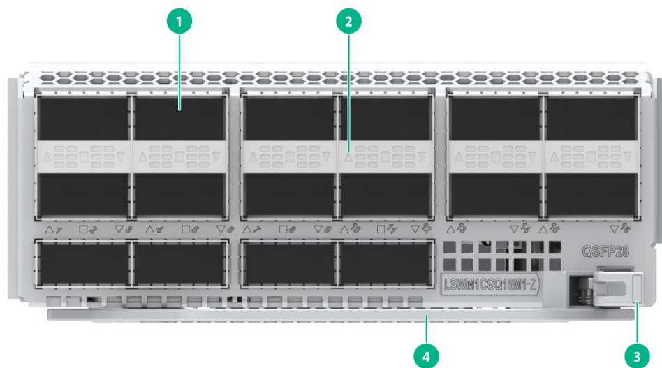
图4-2 LSWM1CGQ16M1-Z 前面板示意图
