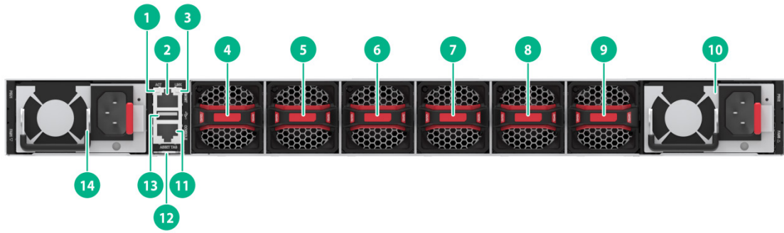
图2-4 S9600XP-24B16DH-G 后面板示意图
