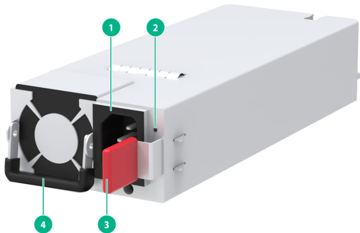
图3-2 PSR1300-12A-C-A-Z 交流电源模块示意图
