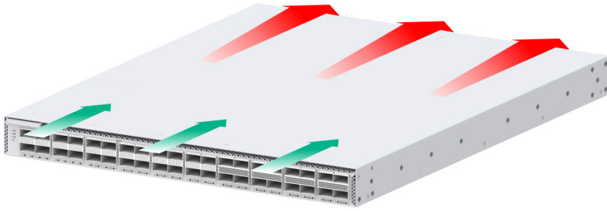
图6-3 端口侧进入电源侧排出散热空气流向示意图（以 S9600XP-8C-G 为例）
