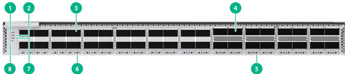
图2-3 S9600XP-24B16DH-G 前面板示意图
